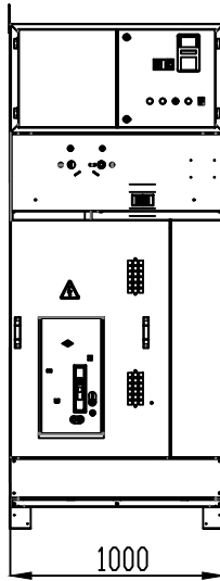
ÖNDEN GÖRÜNÜŞ FRONT VIEW
