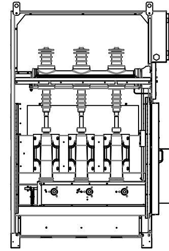
YANDAN GÖRÜNÜŞ LATERAL VIEW
