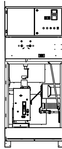
ÖNDEN GÖRÜNÜŞ FRONT VIEW
