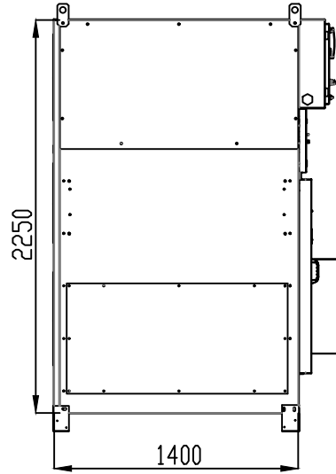
YANDAN GÖRÜNÜŞ LATERAL VIEW
