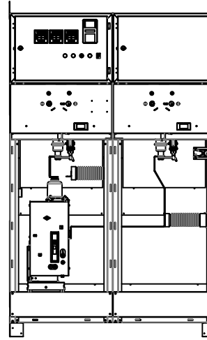
ÖNDEN GÖRÜNÜŞ FRONT VIEW
