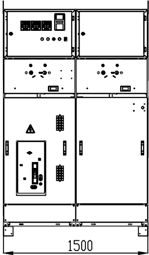
ÖNDEN GÖRÜNÜŞ FRONT VIEW
